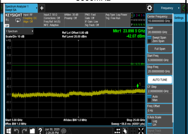
802.11b,2437MHz,Ant1,Plot 5,5000MHz~25000MHz
