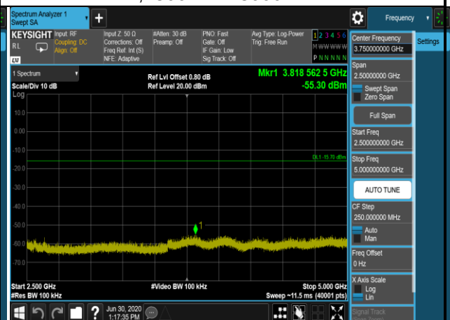
802.11n(HT20),2412MHz,Ant1,Plot 4,2500MHz~5000MHz
