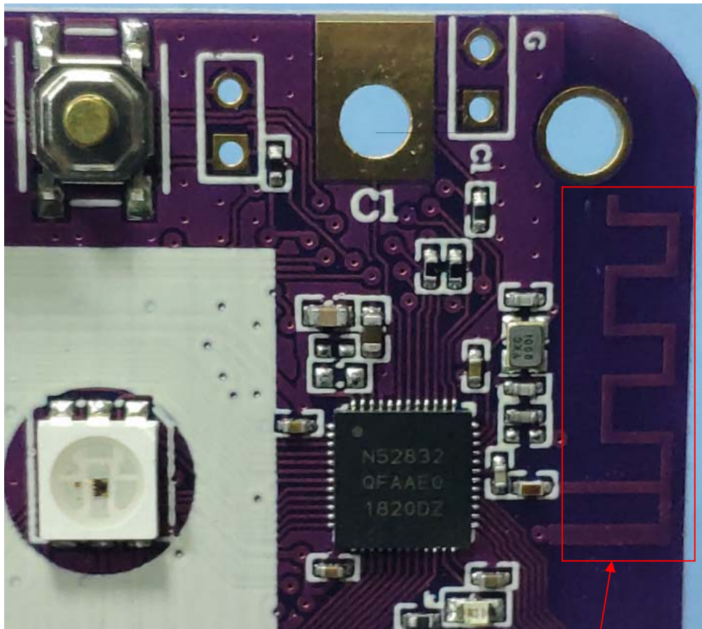
2.4G Antenna
