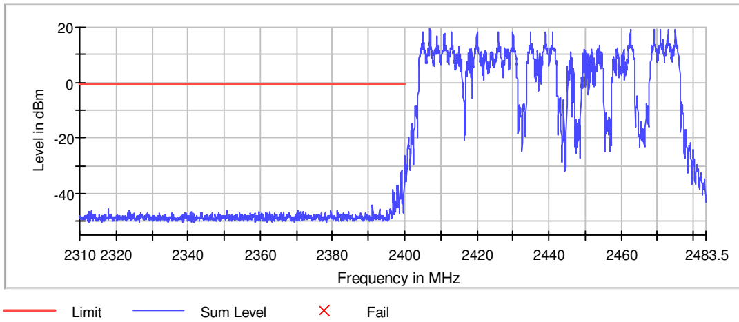
Band Edge
