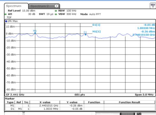
\Pi/4 -DQPSK
