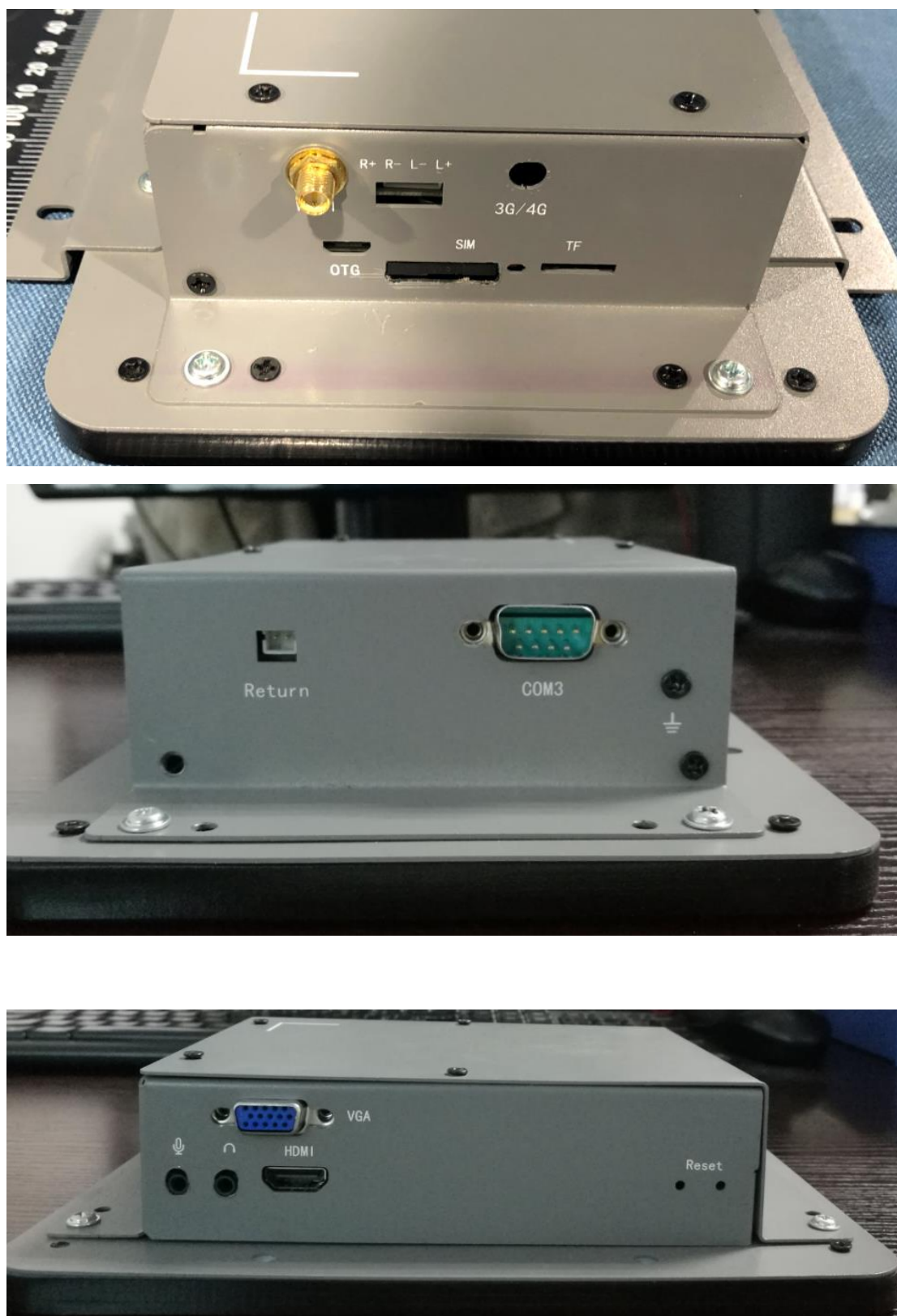
图 1.1: A9 工控机 7 寸一体机外观图
