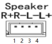
图 2.4 Speaker 端口图
