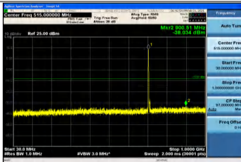
Band17-5MHz-QPSK-23825-1RB#0-Range2:100~5000MHz
