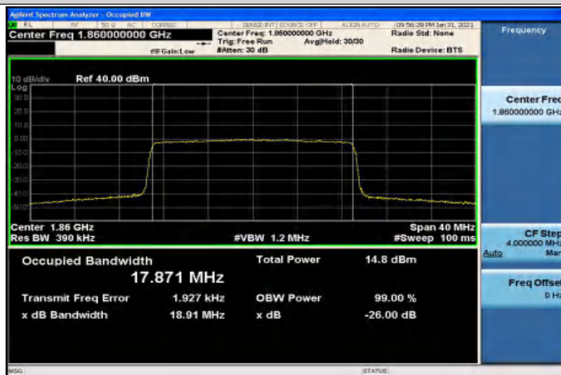
Band2-20MHz-16QAM-18900-100RB#0-18.016
