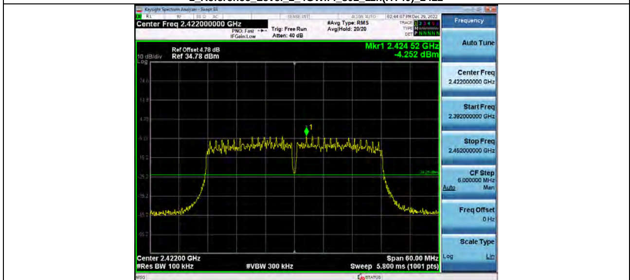
2_Bandedge_2_4GWiFi_NVNT_ANT2_802_11n(HT40) 2422
