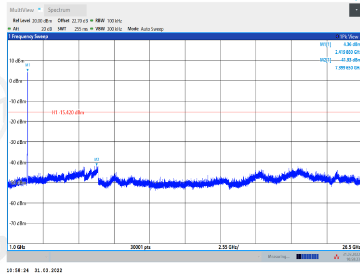
11N20MIMO_Ant2_2412_0~Reference
