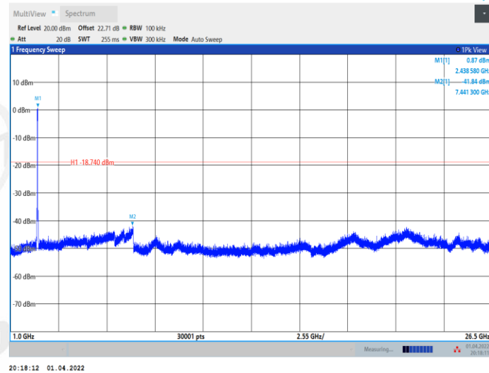
11N40MIMO_Ant2_2422_0~Reference
