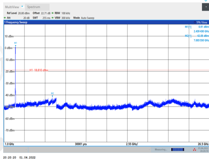
11N40MIMO_Ant1_2437_0~Reference
