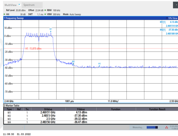
11N20MIMO_Ant2_High_2462
