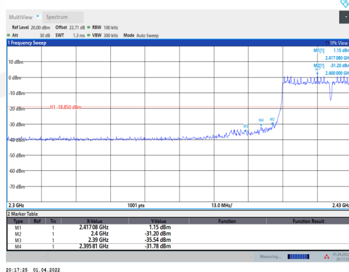
11N40MIMO_Ant2_Low_2422
