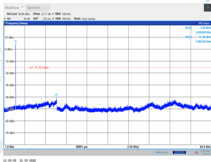
11N20MIMO_Ant2_2437_0~Reference
