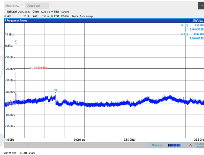
11N40MIMO_Ant2_2452_0~Reference
