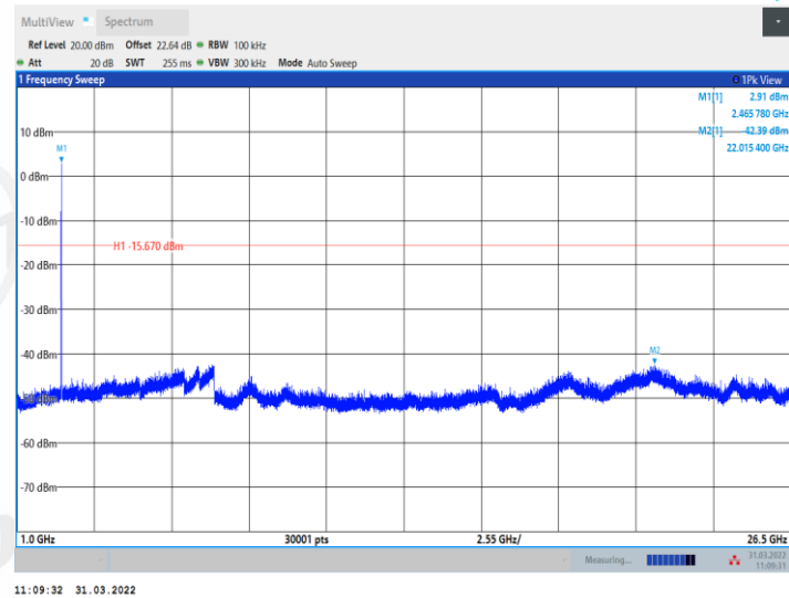
11N20MIMO_Ant2_2462_0~Reference
