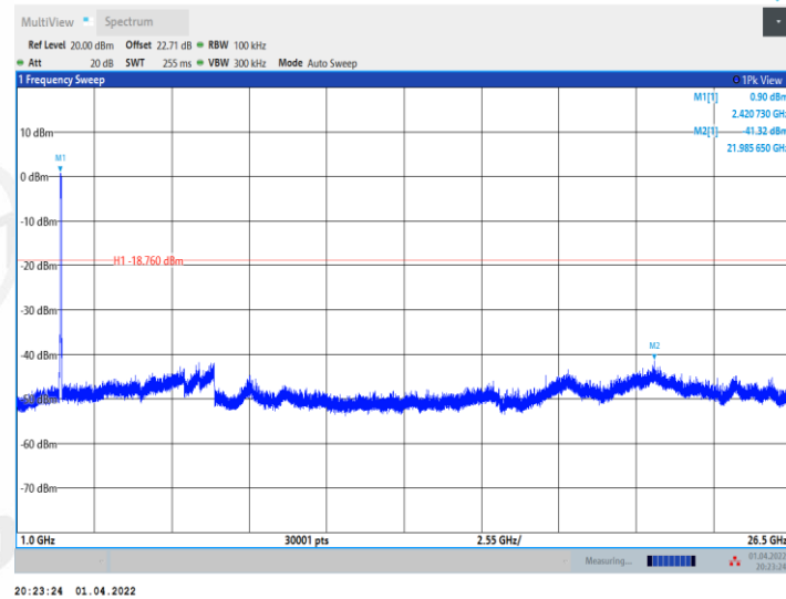
11N40MIMO_Ant2_2437_0~Reference
