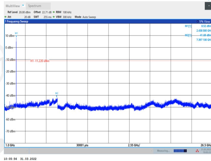
11B_Ant2_2437_0~Reference
