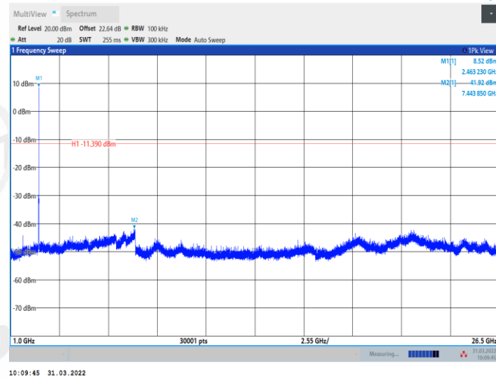
11B_Ant2_2462_0~Reference
