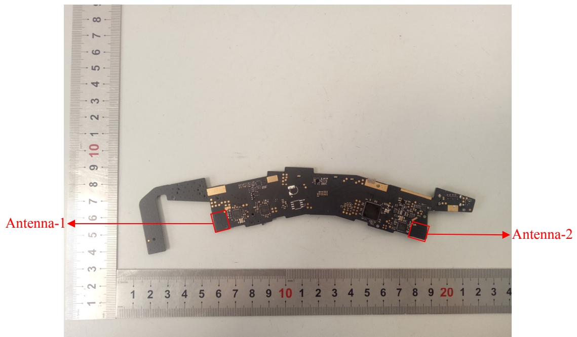
EUT – PCB-1 Bottom ChipView-1
