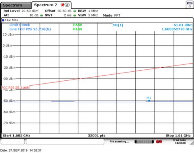
Figure 8.6-1: L. channel (QPSK)
