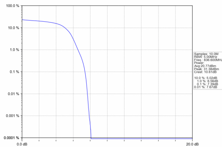
Band5_HSUPA_MCH_836.6MHz_Subtest 1_NTNV
