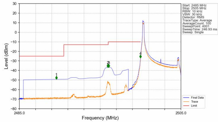
Band7_5MHz_QPSK_LCH_2502.5MHz_RB_1_0_NTNV
