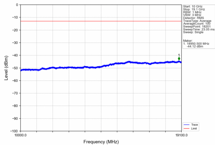
Band2_15MHz_QPSK_MCH_1880MHz_RB_1_0_NTNV
