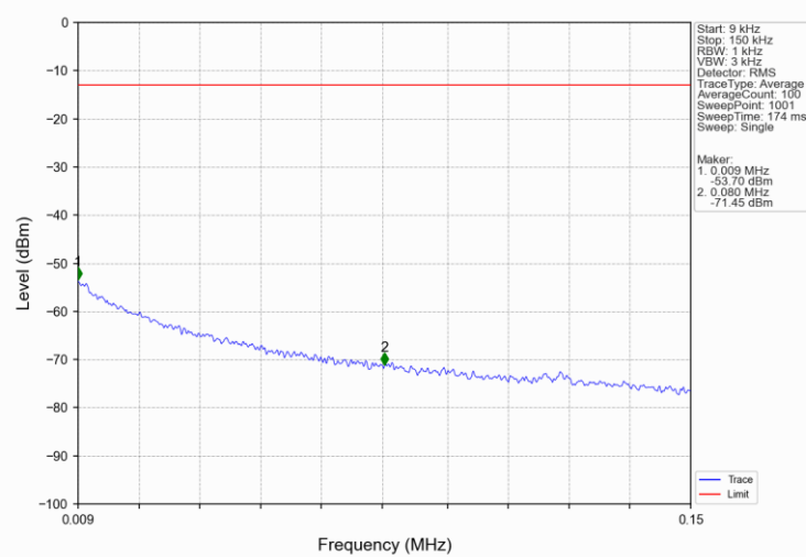
Band2_15MHz_QPSK_LCH_1857.5MHz_RB_1_0_NTNV
