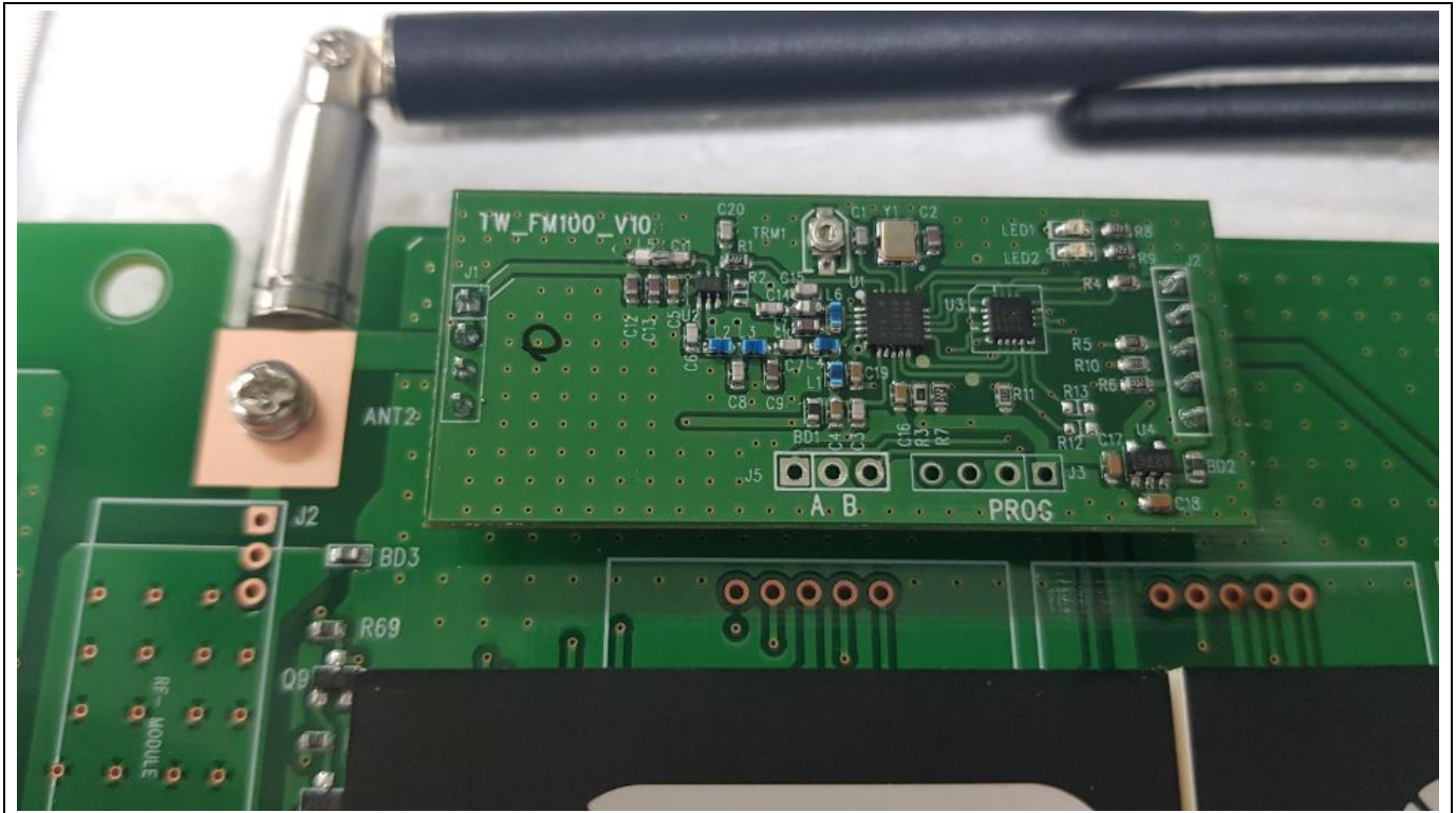
<RX Module>
