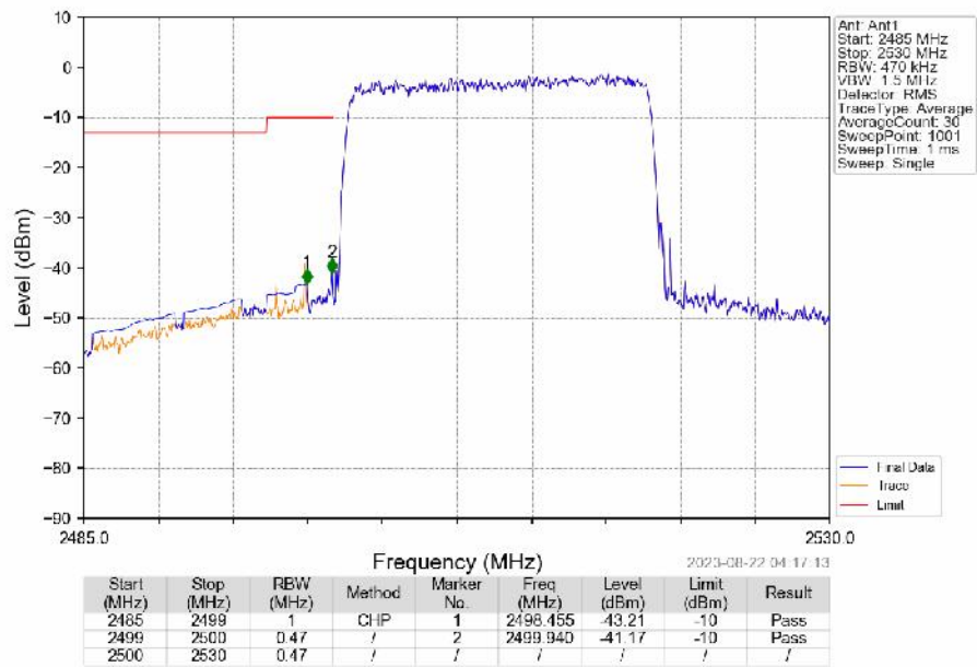
Band7_20MHz_16QAM_LCH_2510MHz_RB_100_0_NTNV
