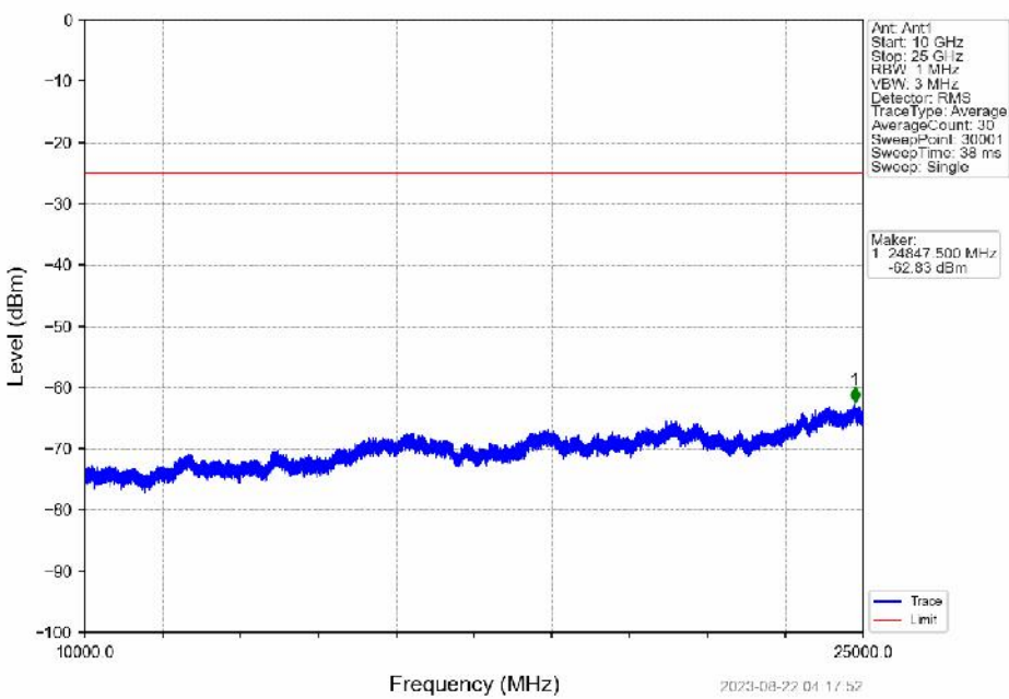
Band7_20MHz_16QAM_MCH_2535MHz_RB_1_0_NTNV
