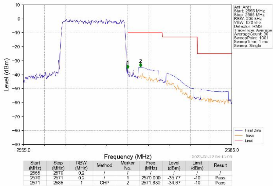
Band7_10MHz_QPSK_HCH_2565MHz_RB_1_49_NTNV
