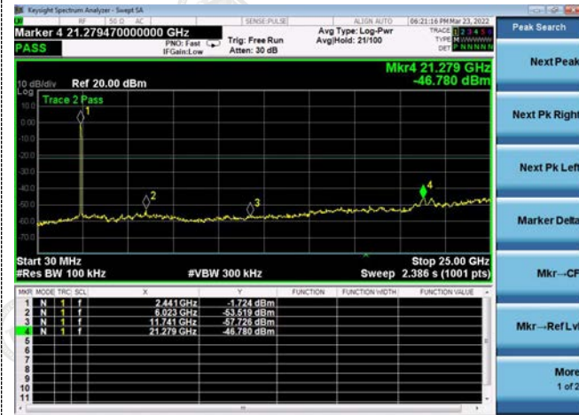
30MHz-25G
