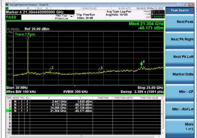
30MHz-25G
