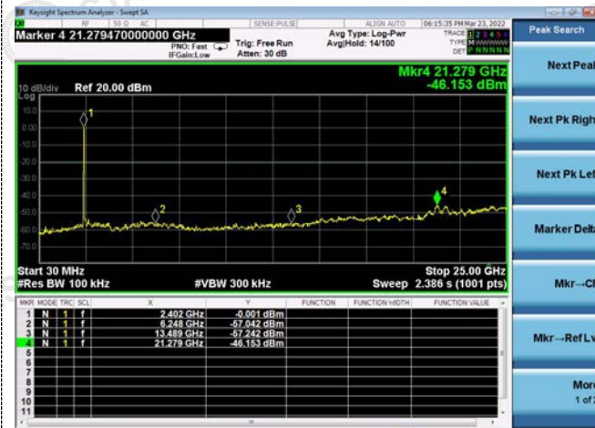
30MHz-25G
