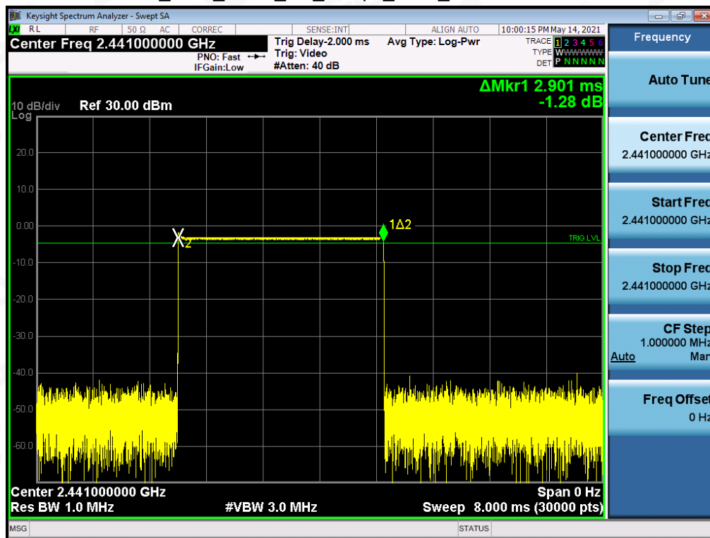
BR_HOP_ANT1_NA_1Mbps_2441_Time per Burst
