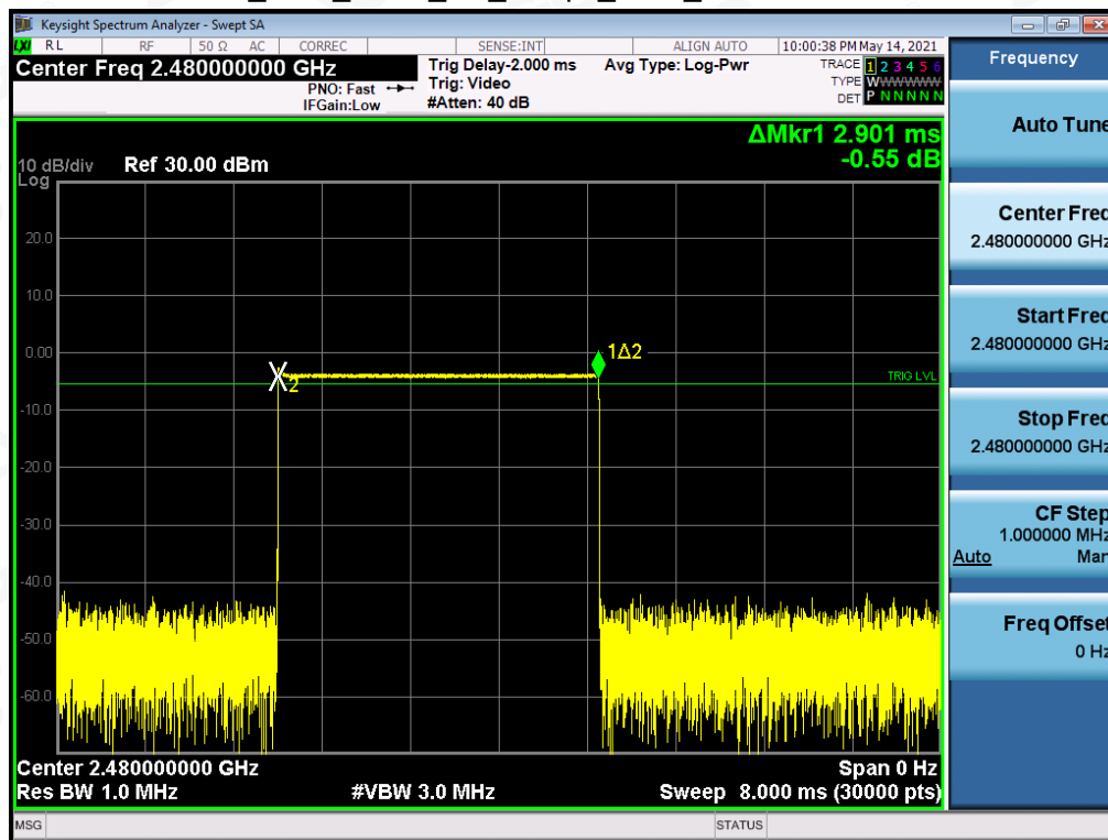
BR_HOP_ANT1_NA_1Mbps_2480_Time per Burst
