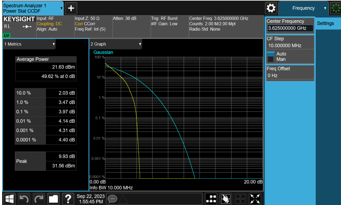
Plot 7-54. PAR Plot (NR Band n78 - 10MHz DFT-s-OFDM BPSK- Full RB)
