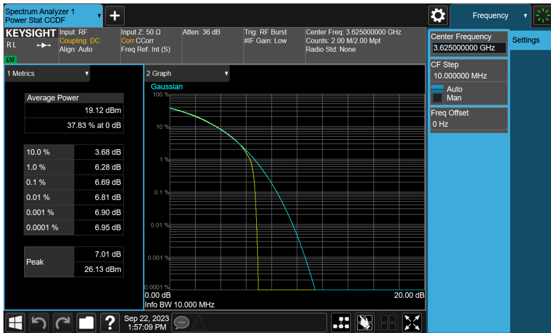
Plot 7-55. PAR Plot (NR Band n78 - 10MHz CP-OFDM QPSK- Full RB)
