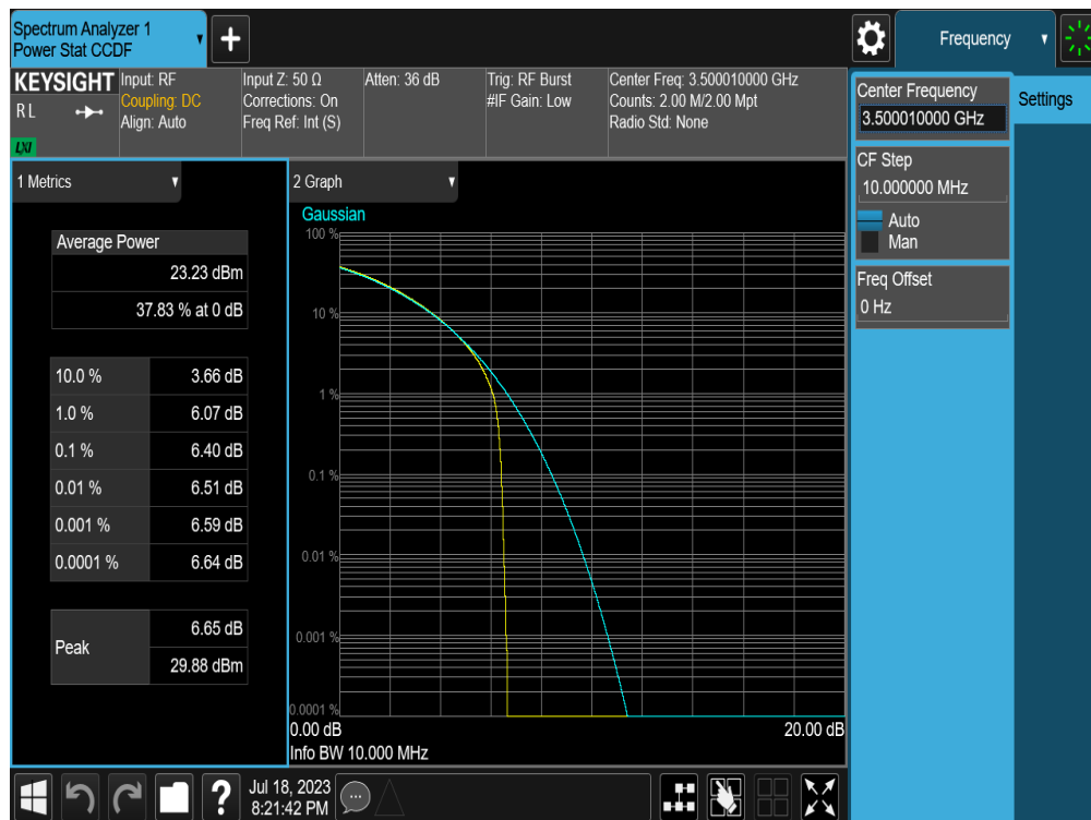
Plot 7-50. PAR Plot (NR Band n78 - 10MHz CP-OFDM QPSK-Full RB)
