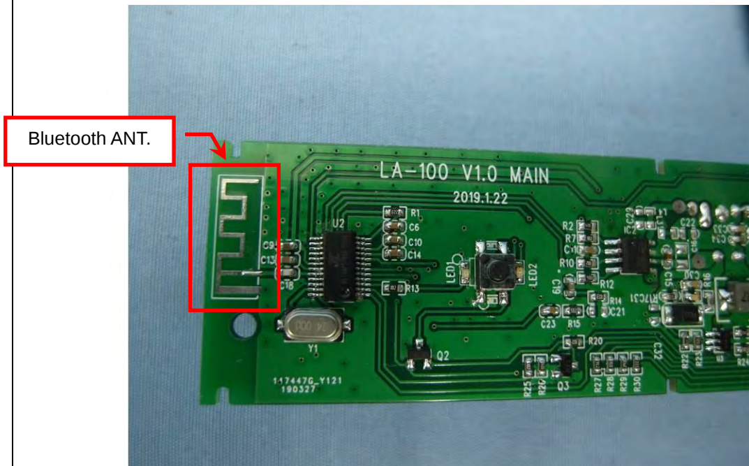
EUT Photo (6)
