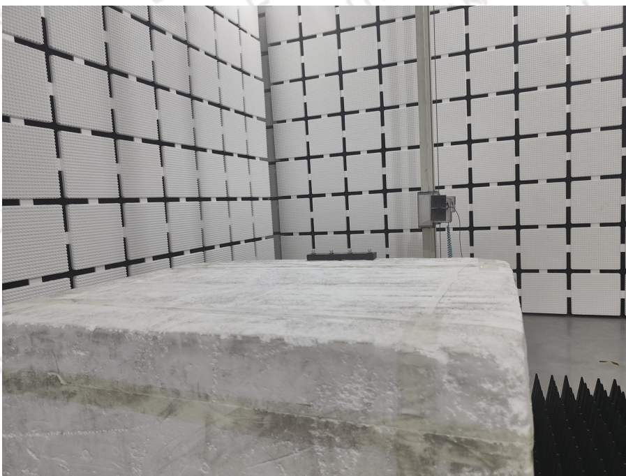
30MHz-1000MHz
