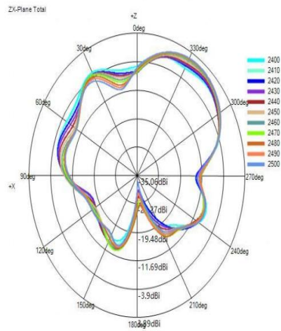
(1) X-Z 面(单位: dBi):
