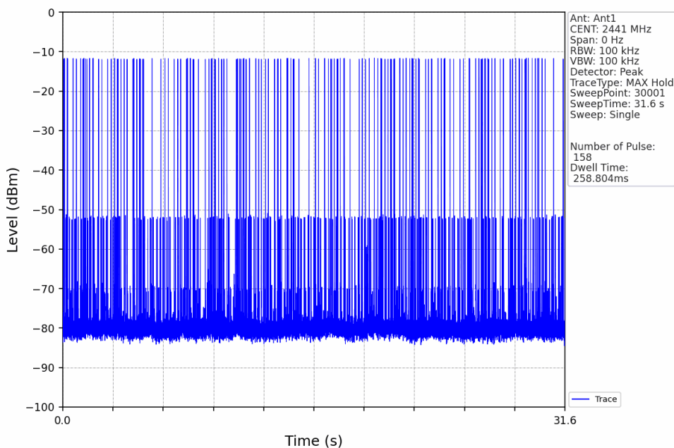
GFSK_DH3_HOPP_Ant1_NTNV
