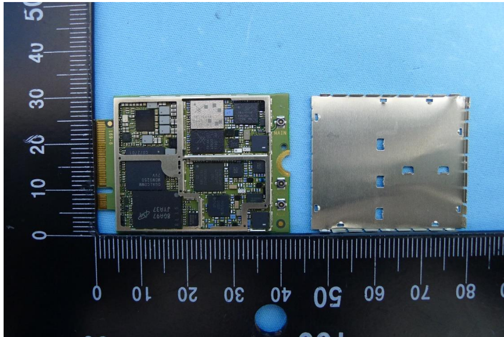
(66) RF Module (SIERRA EM7565)
