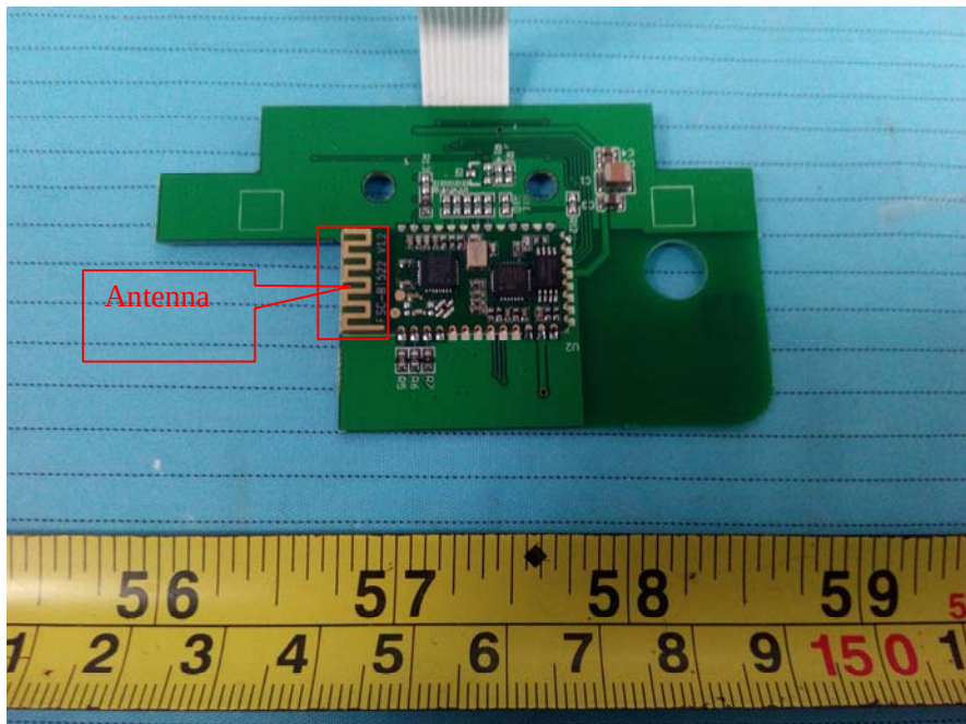
EUT – Mian Board 1 Top View
