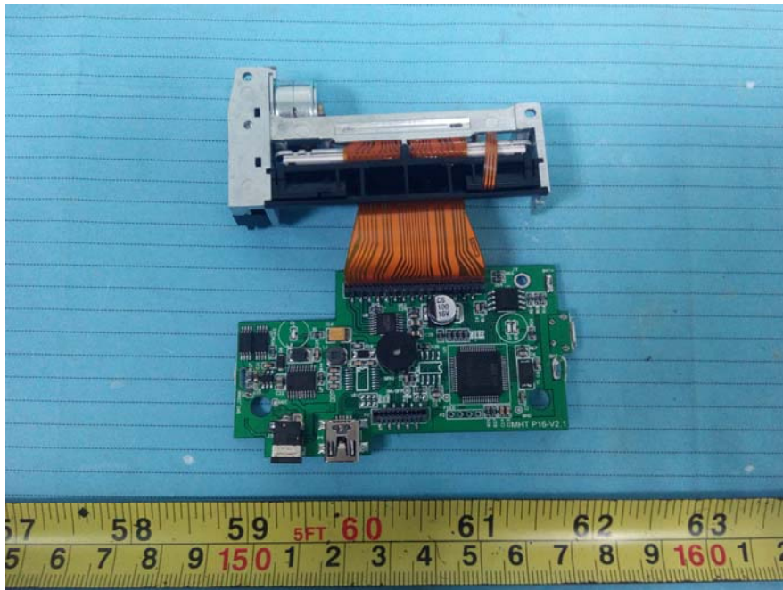
EUT – Mian Board 2 Top View
