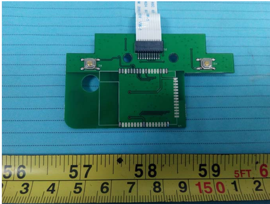
EUT – Mian Board 1 Bottom View
