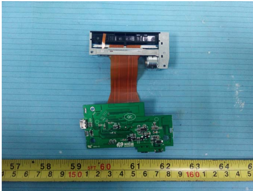
EUT – Mian Board 2 Bottom View
