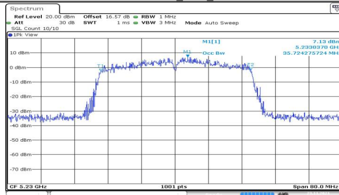
11N40MIMO_Ant1_5230
