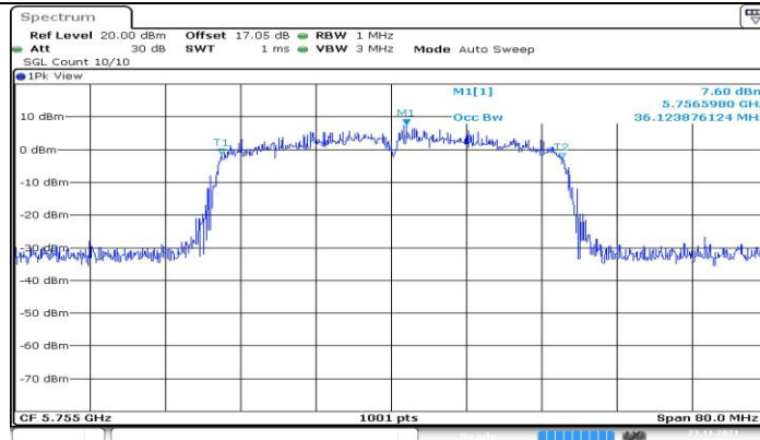
11N40MIMO_Ant2_5755
