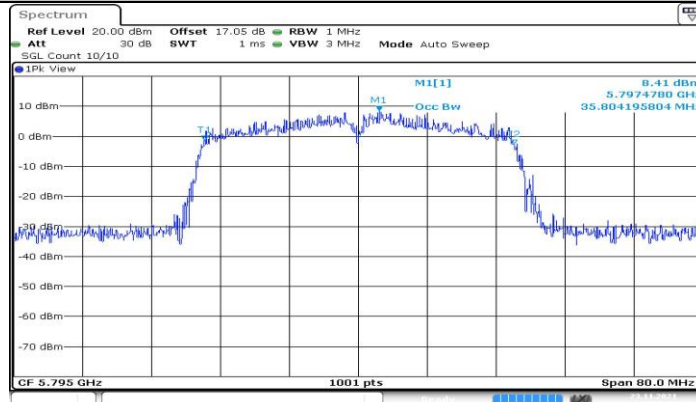
11N40MIMO_Ant1_5795
