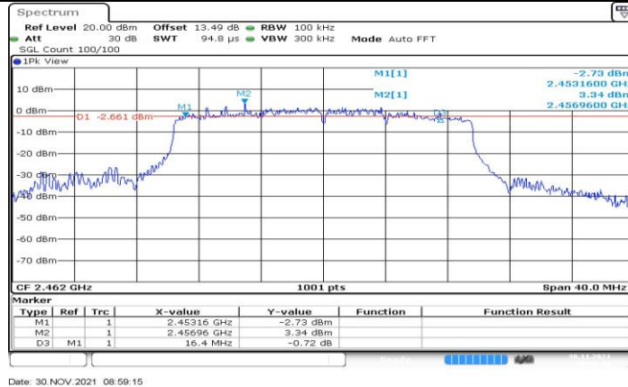
11AX20MIMO_Ant2_2462
