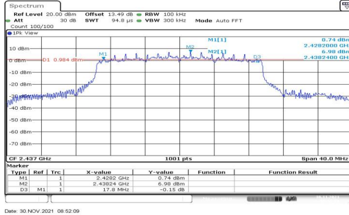
11AX20MIMO_Ant1_2437
