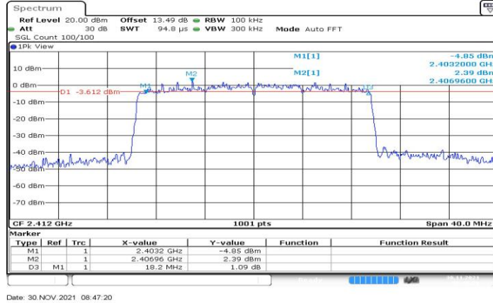
11AX20MIMO_Ant2_2412
