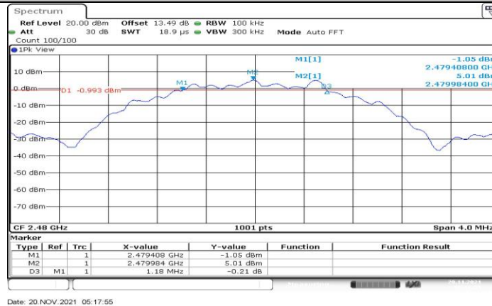
BLE_2M_Ant1_2480
