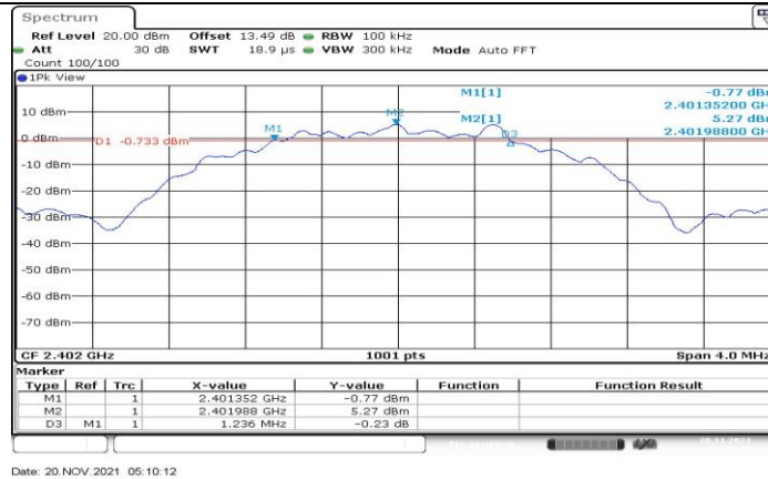
BLE_2M_Ant1_2402
