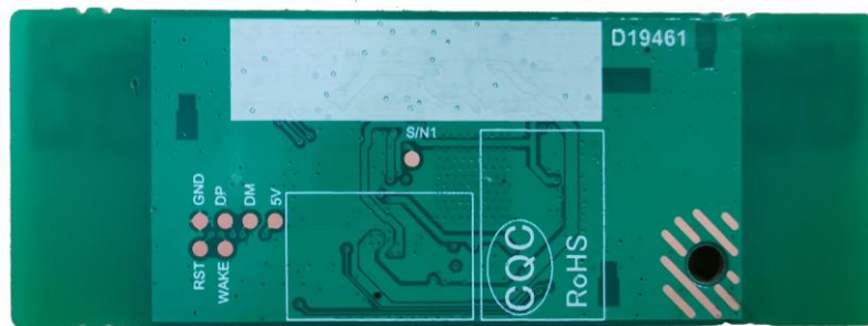
背视图 ( bottom view )
