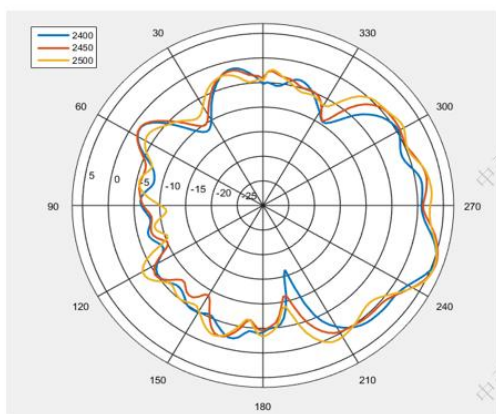
XOY面 ( \theta=90^\circ )
