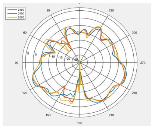
XOZ面 ( \phi=0^\circ )
