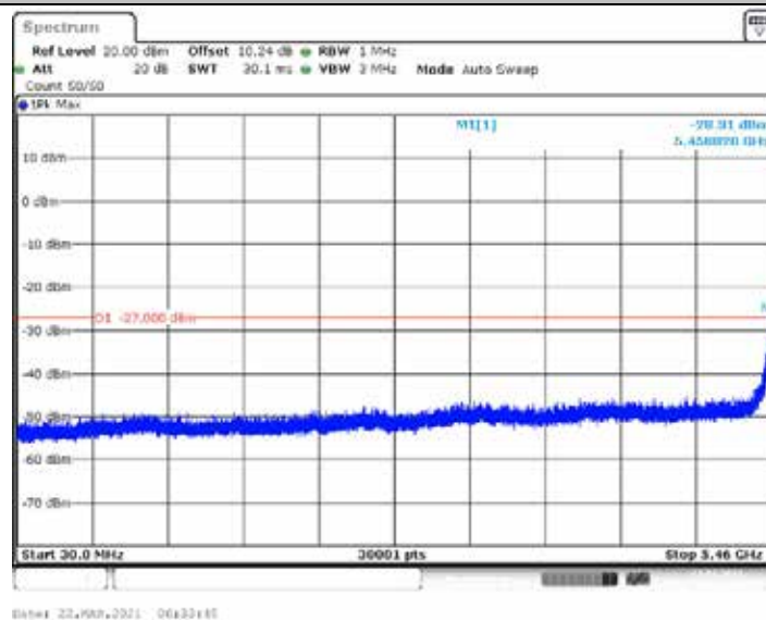
11AX40MIMO_Ant2_5510_30~5460
