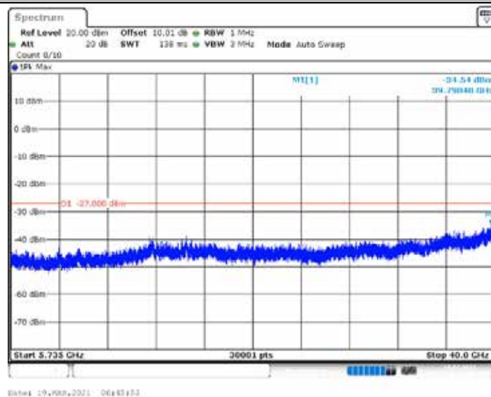
11N40MIMO_Ant1_5550_5735~40000
