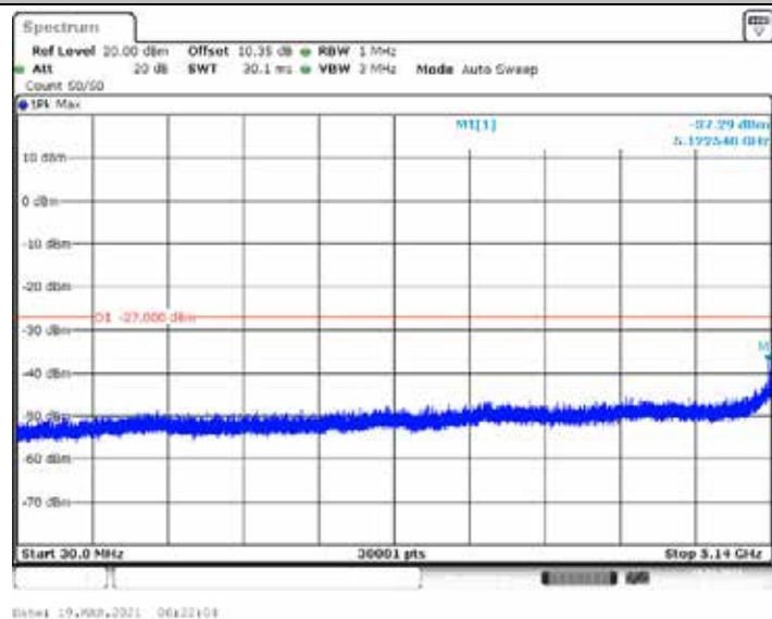
11N40MIMO_Ant2_5230_30~5140
