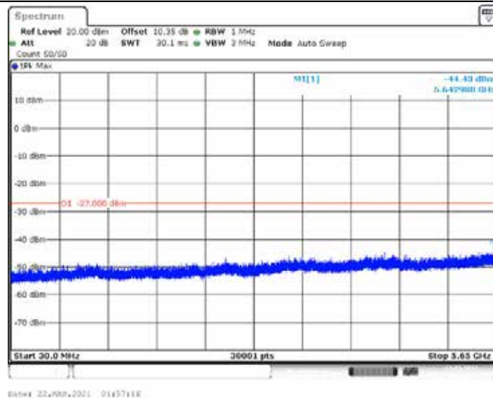
11AX20MIMO_Ant2_5825_30~5650
