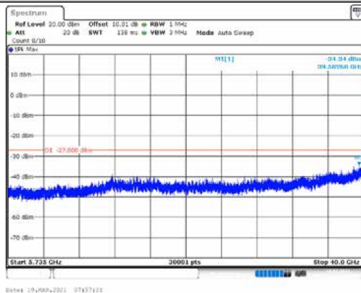
11AC20MIMO_Ant1_5500_5735~40000
