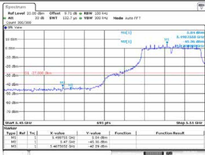
11AC20ISO_Ant1_Low_5500
