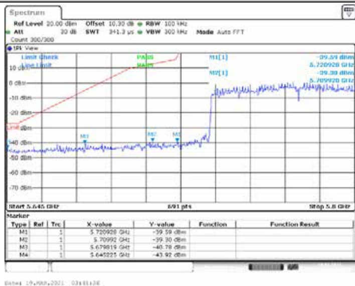
11AX80ISO_Ant2_Low_5775
