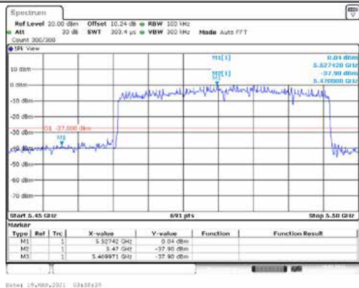
11AX80ISO_Ant2_Low_5530
