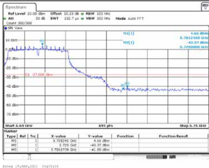
11N20MIMO_Ant2_High_5700
