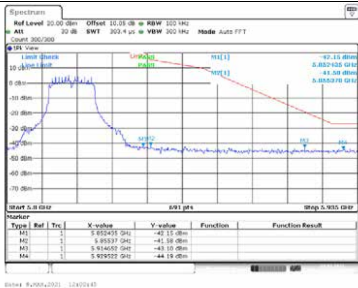
11N40ISO_Ant1_Low_5755
