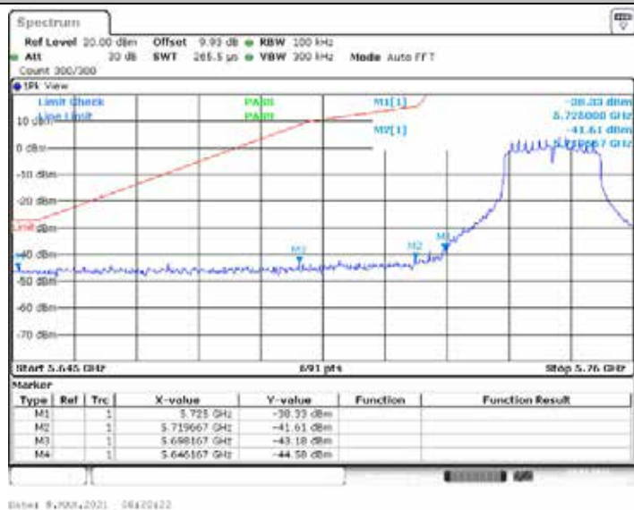
11N20ISO_Ant1_Low_5745
