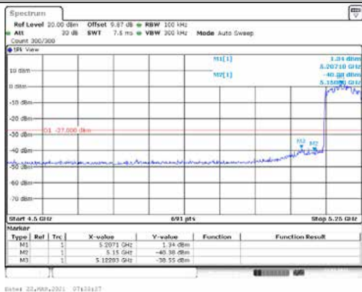
11AX80MIMO_Ant2_Low_5210
