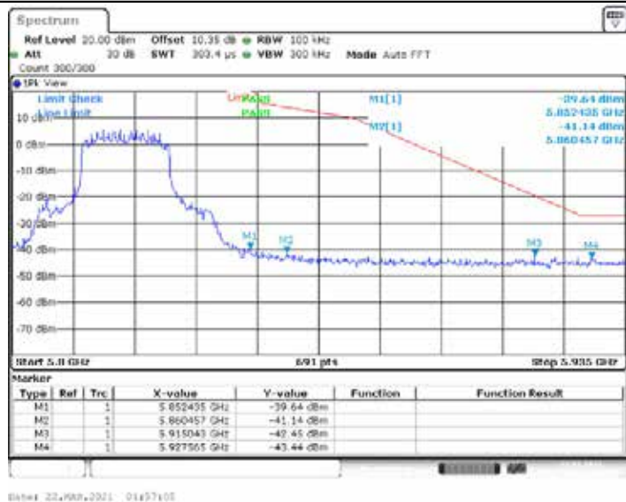
11AX20MIMO_Ant2_High_5825
