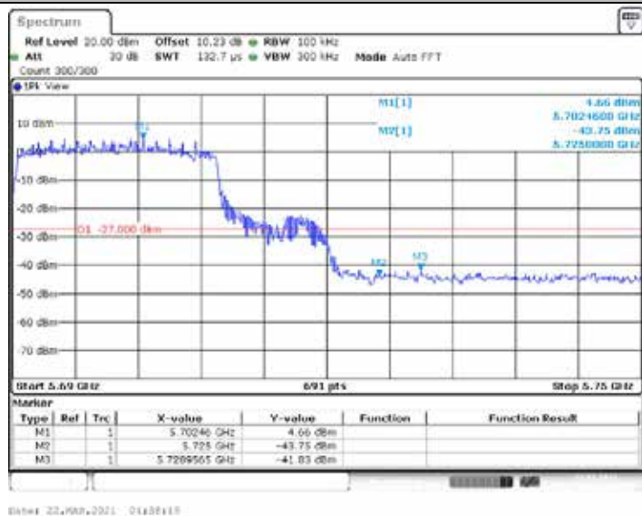
11AX20MIMO_Ant2_High_5700
