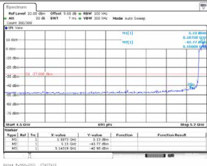
11AC40ISO_Ant2_Low_5190
