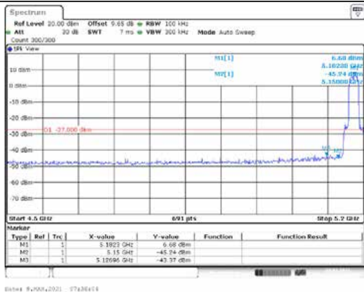
11AX20ISO_Ant2_Low_5180
