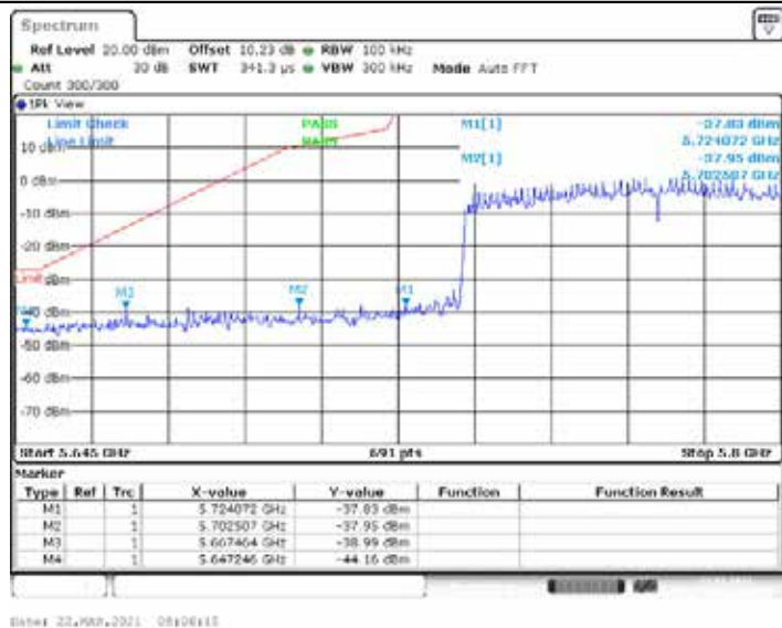
11AX80MIMO_Ant1_Low_5775
