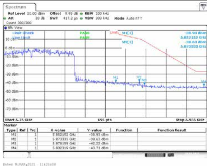
11AX80ISO_Ant2_Low_5775
