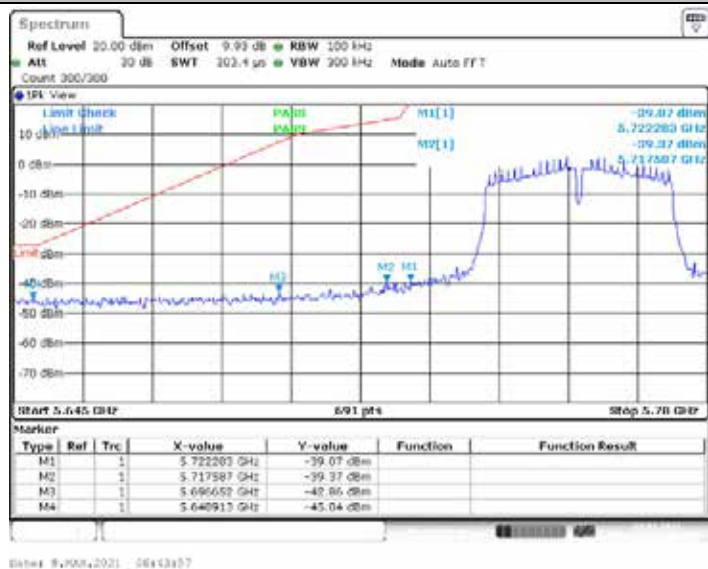
11N40ISO_Ant2_Low_5755
