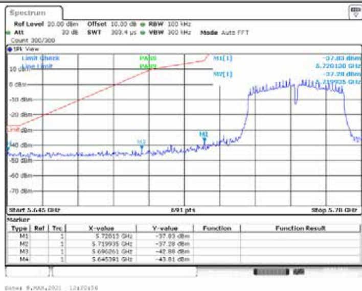
11N40ISO_Ant2_Low_5755
