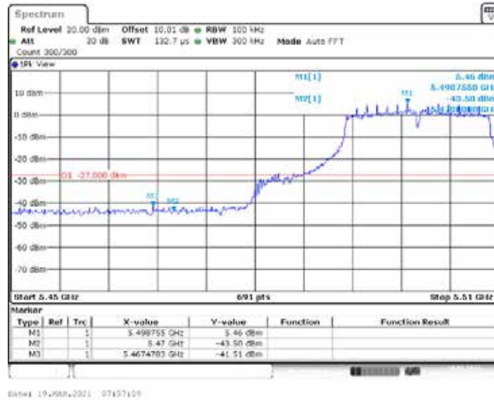
11AC20MIMO_Ant2_Low_5500
