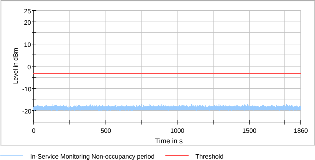
IEEE 802.11a 5260MHz
