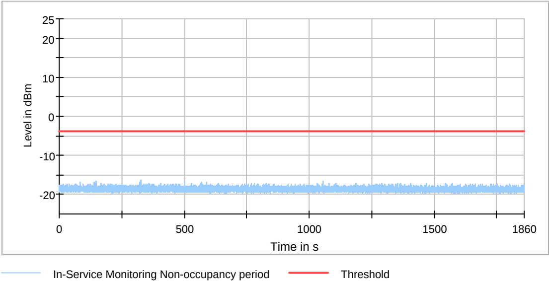
IEEE 802.11ac VHT80 5290MHz
