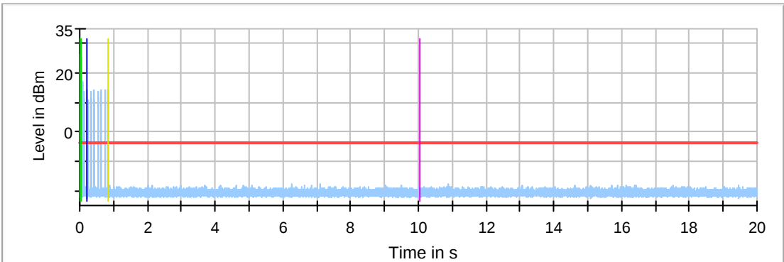
IEEE 802.11n HT40 5270MHz
