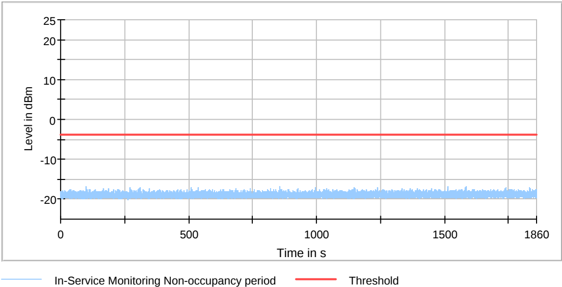
IEEE 802.11n HT40 5270MHz
