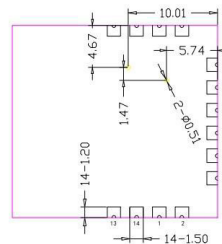
模组底视图
