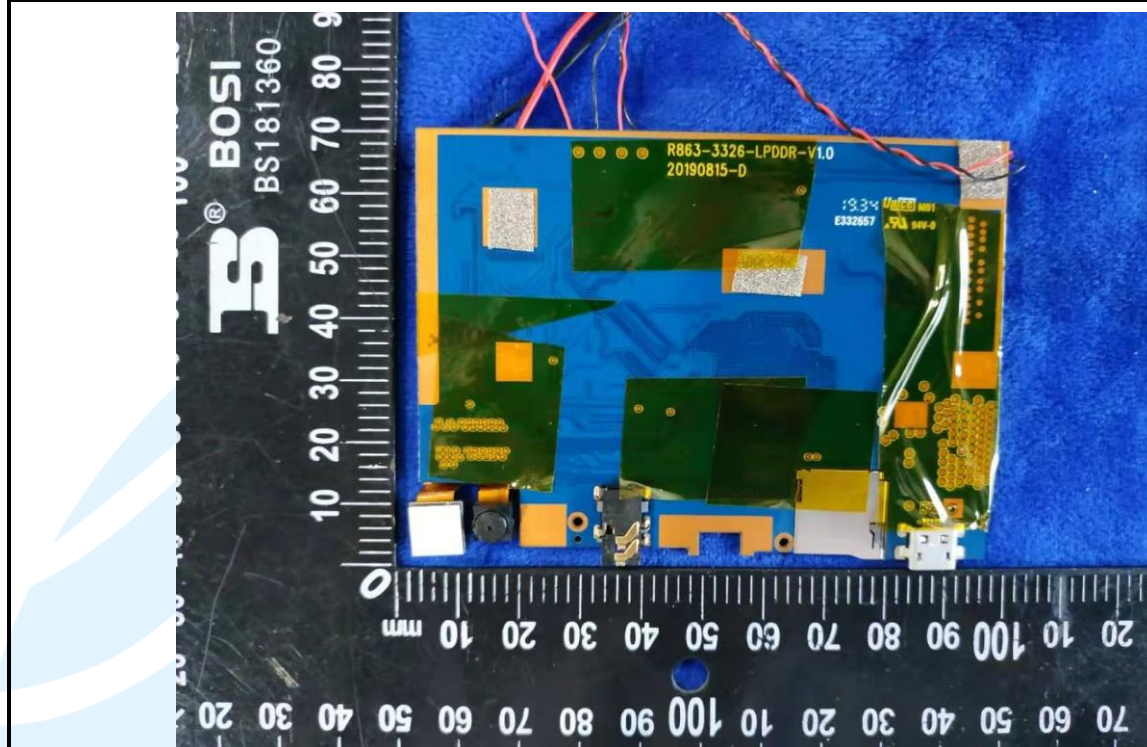
EUT Photo
