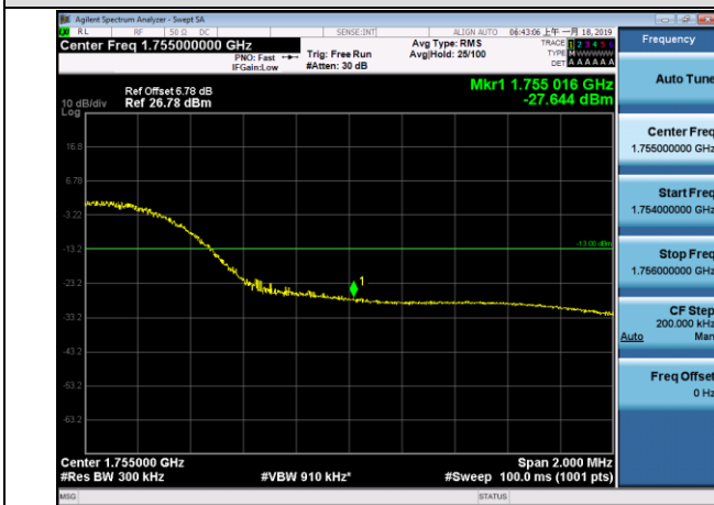
HCH_QPSK_75RB#0
