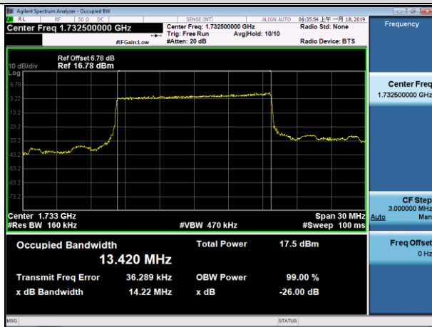
MCH_QPSK_75RB#0
