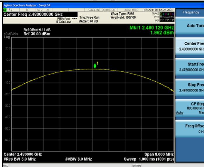
DH5_Ant2_2480
