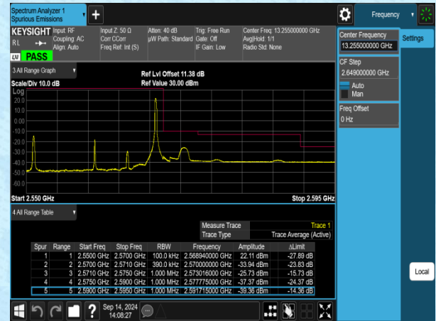
Band7-20MHz-QPSK-21350-1RB#99-PASS
