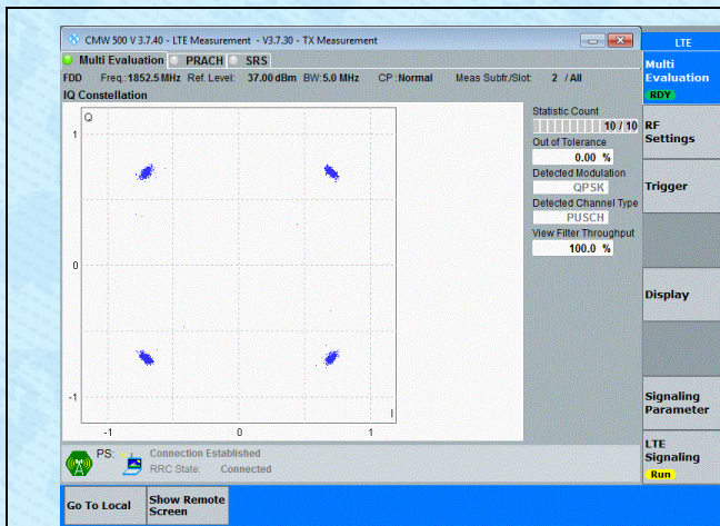
Band2-5MHz-QPSK-18625-25RB#0-PASS
