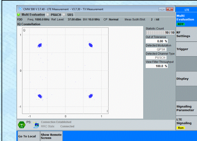
Band2-10MHz-QPSK-18900-50RB#0-PASS
