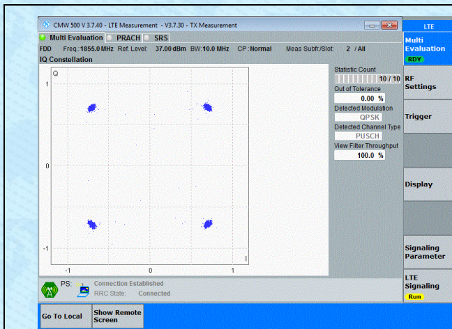
Band2-10MHz-QPSK-18650-50RB#0-PASS
