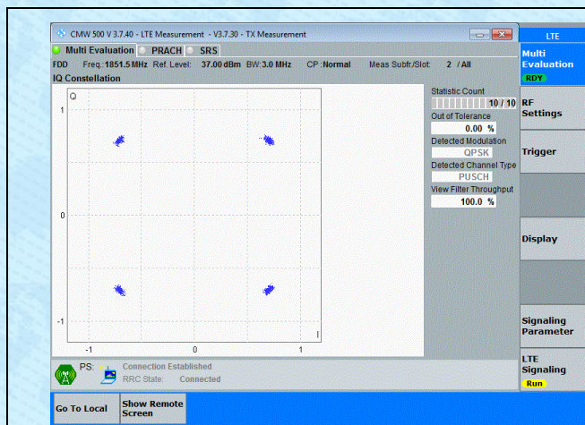
Band2-3MHz-QPSK-18615-15RB#0-PASS
