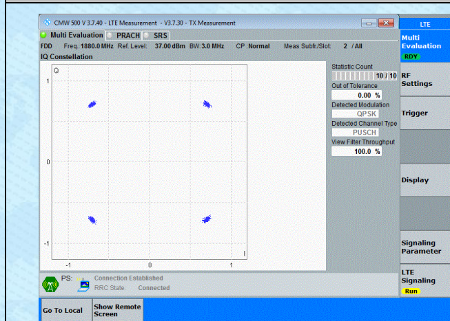
Band2-3MHz-QPSK-18900-15RB#0-PASS
