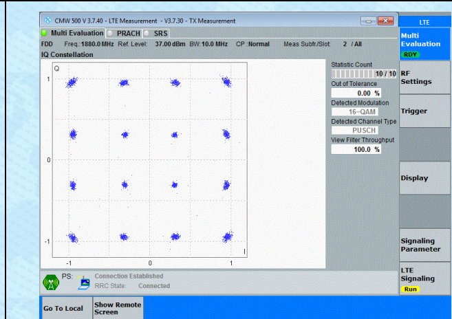
Band2-10MHz-16QAM-18900-50RB#0-PASS
