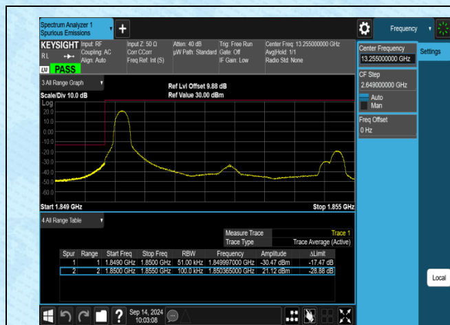
Band2-5MHz-16QAM-18625-1RB#0-PASS
