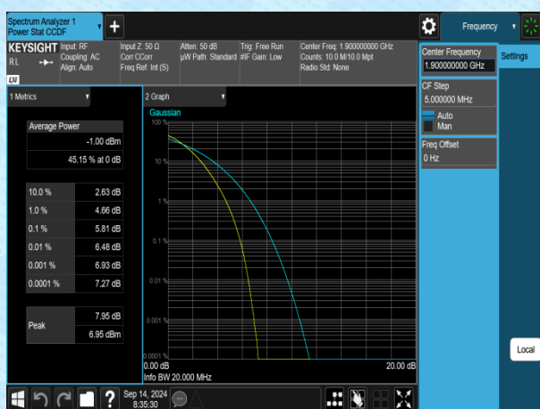
Band2-20MHz-QPSK-19100-1RB#0-PASS
