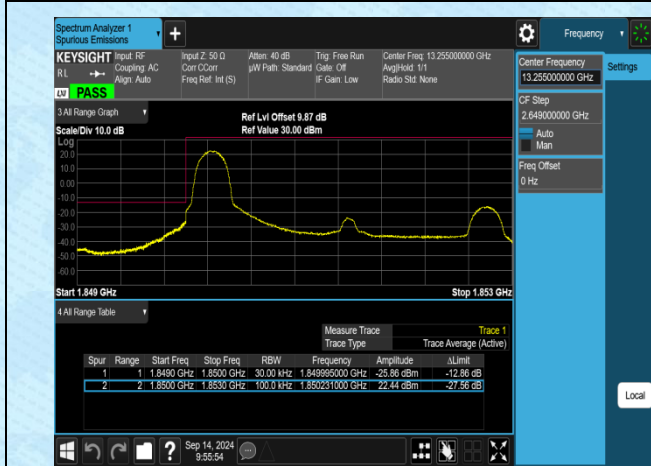
Band2-3MHz-QPSK-18615-1RB#0-PASS
