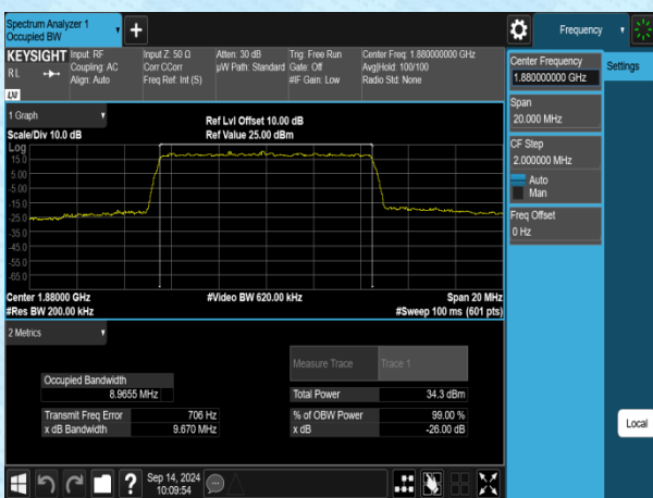
Band2-10MHz-QPSK-18900-50RB#0-PASS
