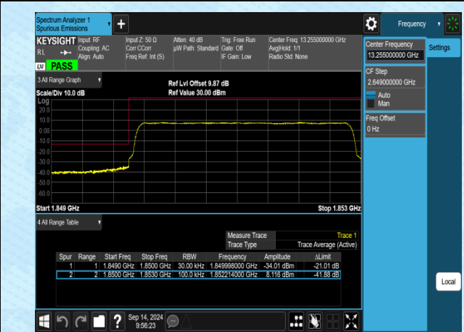
Band2-3MHz-QPSK-18615-15RB#0-PASS
