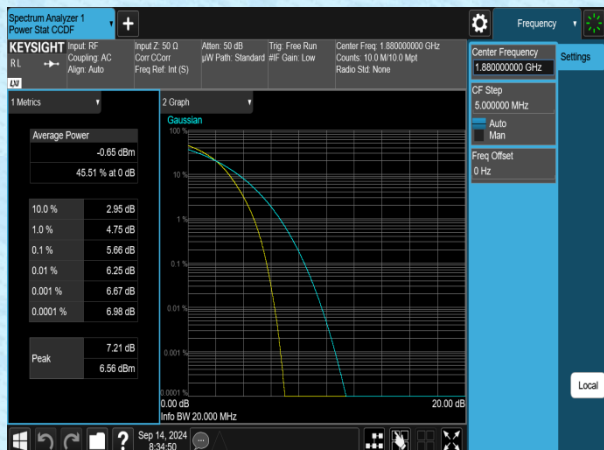
Band2-20MHz-16QAM-18900-1RB#0-PASS
