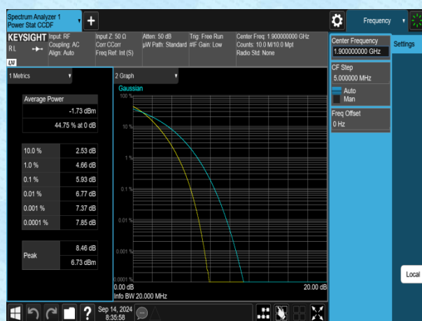
Band2-20MHz-QPSK-19100-100RB#0-PASS
