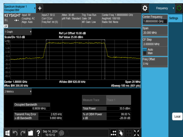
Band2-10MHz-16QAM-18900-50RB#0-PASS
