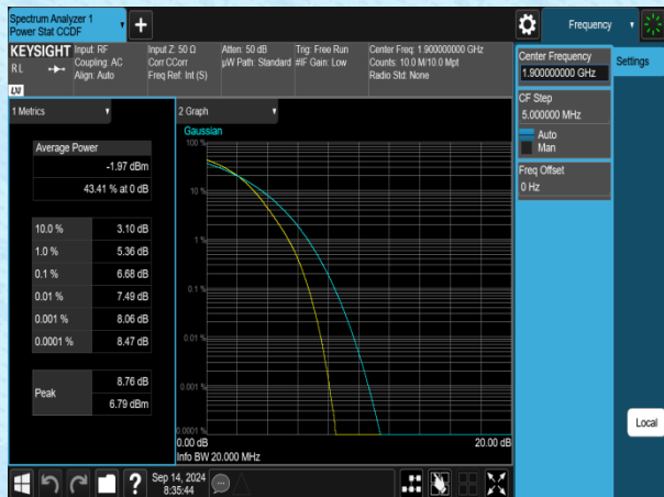
Band2-20MHz-16QAM-19100-1RB#0-PASS
