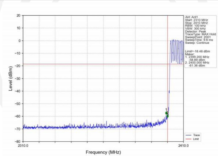
GFSK_DH5_HOPP_Ant1_NTNV
