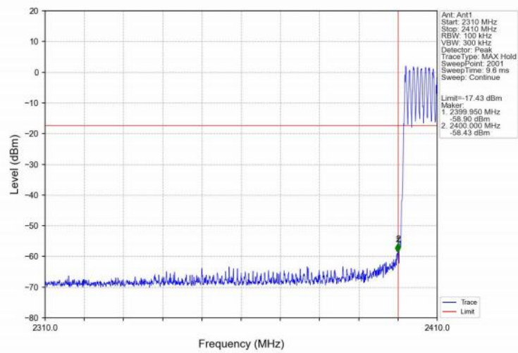
GFSK_DH5_HOPP_2410MHz_Ant1_NTNV
