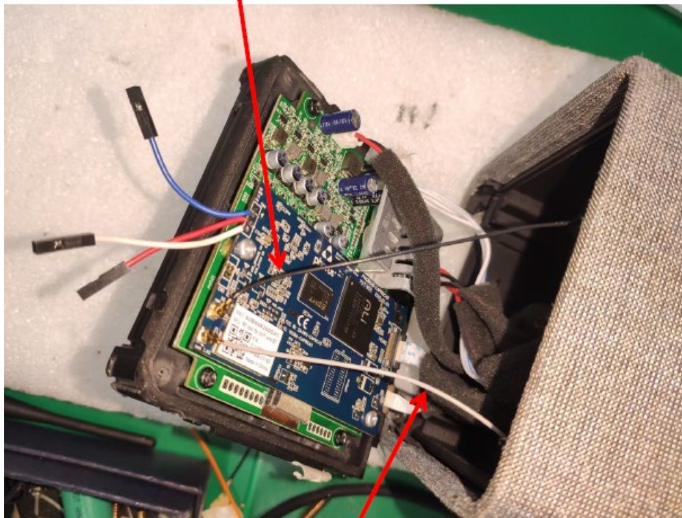
Paly-FI Module 2.4G ANT
