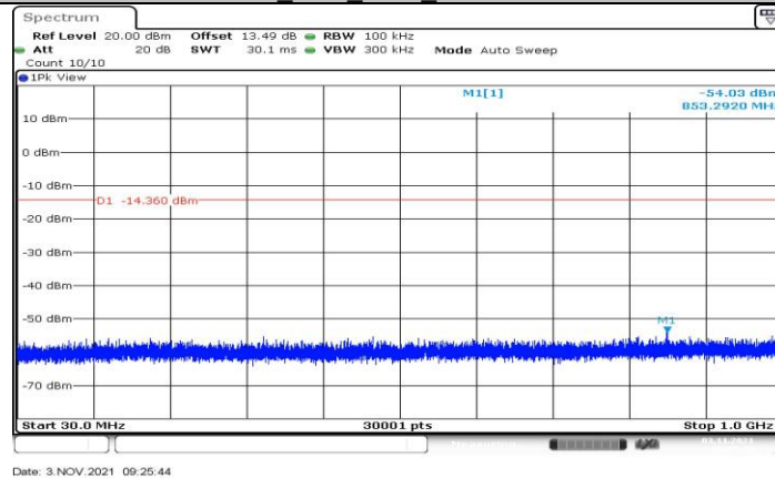
3DH5 Ant1 2441 30~1000
