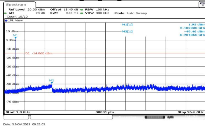
3DH5 Ant1 2402 1000~26500
