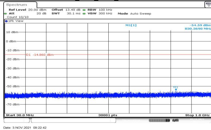
3DH5 Ant1 2402 30~1000
