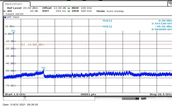
3DH5 Ant1 2441 1000~26500
