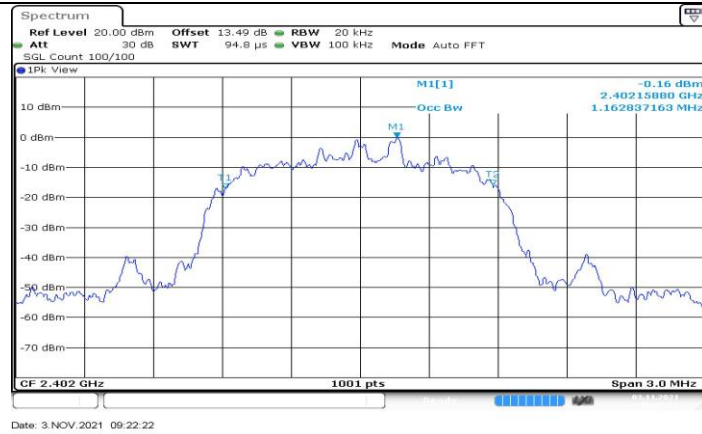
3DH5 Ant1 2402
