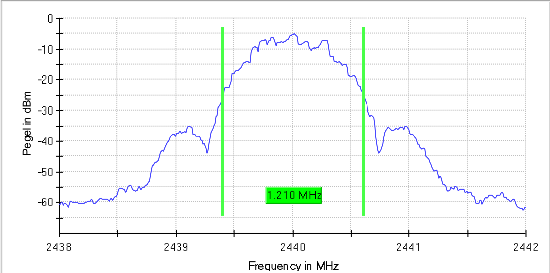
20dB-BW, 2440 MHz, BLE
