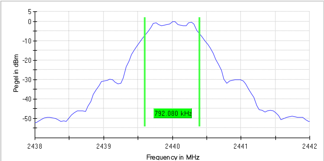
6dB-BW, 2440 MHz, BLE
