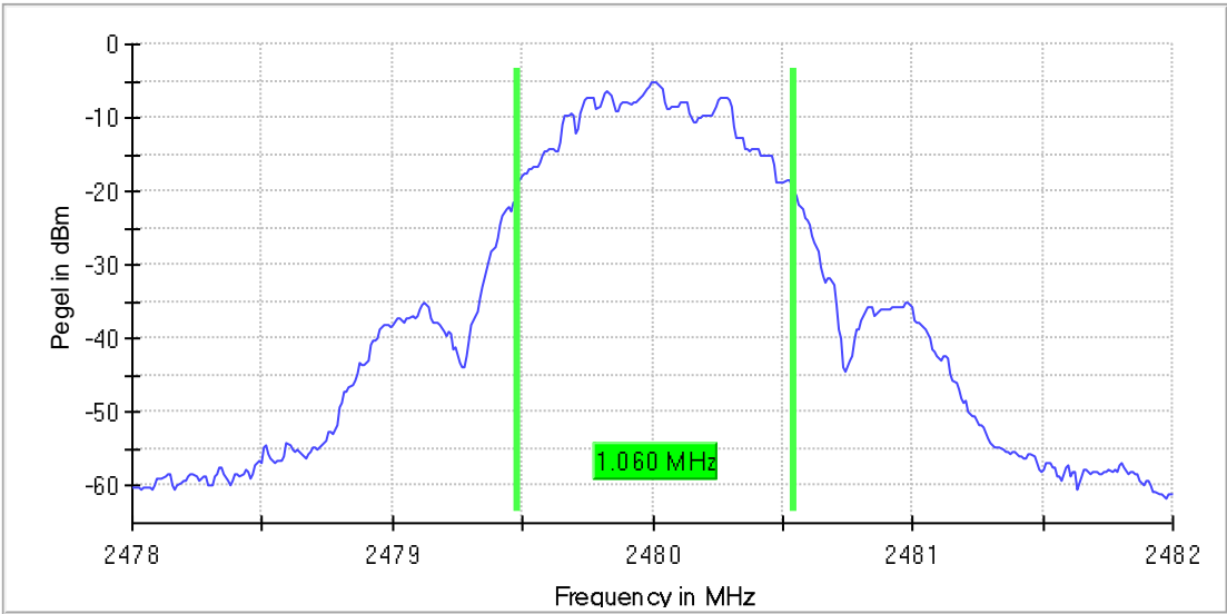
99%-BW, 2480 MHz, BLE
