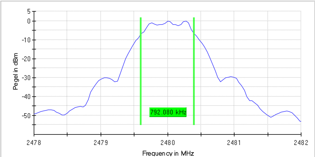
6dB-BW, 2480 MHz, BLE
