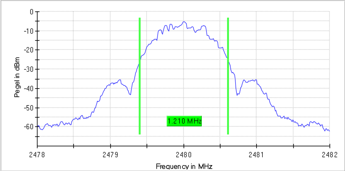
20dB-BW, 2480 MHz, BLE
