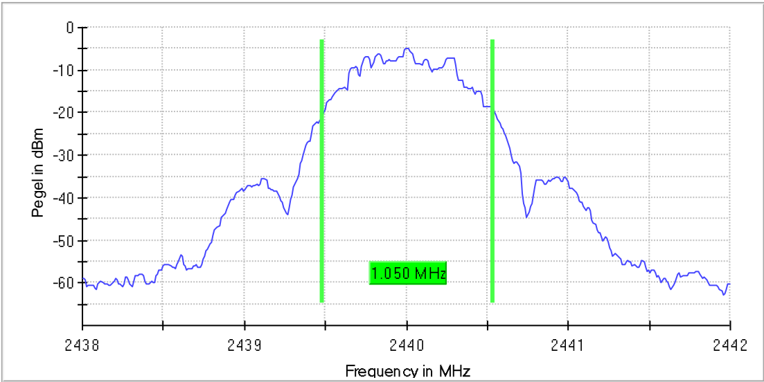
99%-BW, 2440 MHz, BLE
