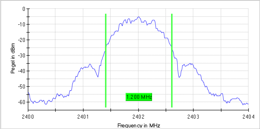
20dB-BW, 2402 MHz, BLE
