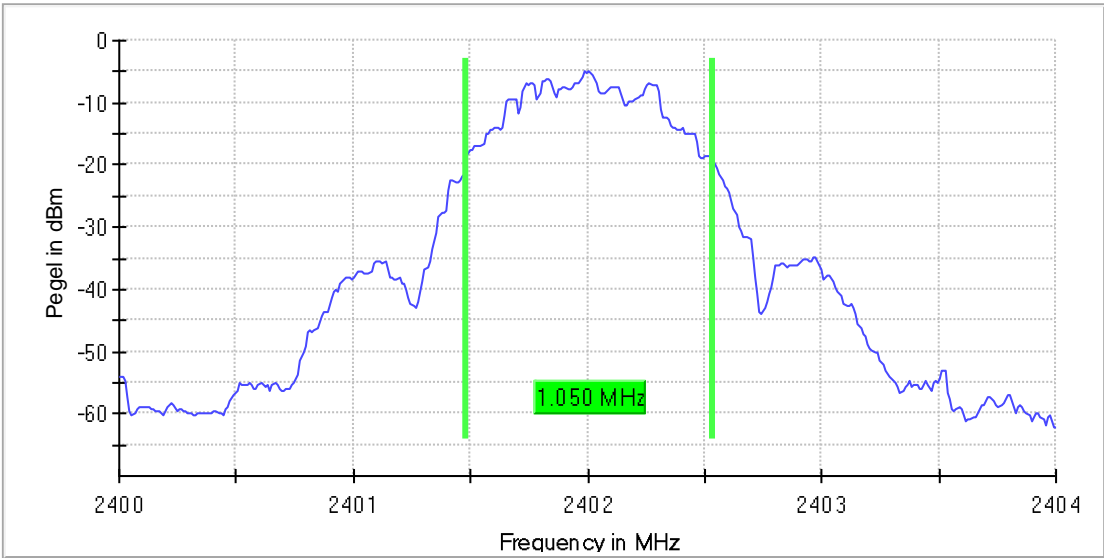
99%-BW, 2402 MHz, BLE
