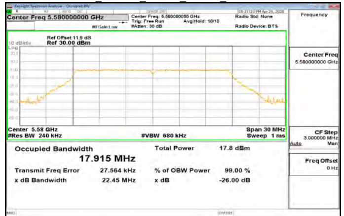
FCC 802.11n 20MHz Chain0 5580MHz
