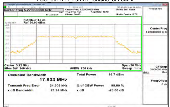
FCC 802.11n 20MHz Chain0 5220MHz
