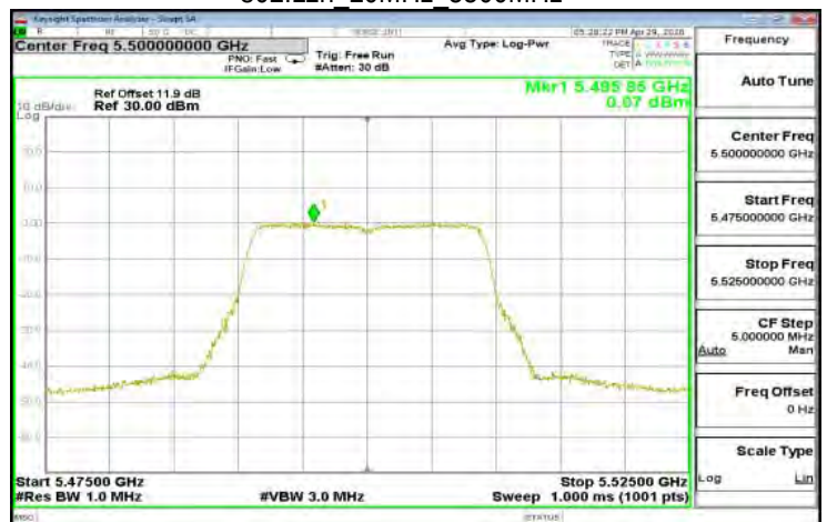
802.11n 20MHz 5500MHz
