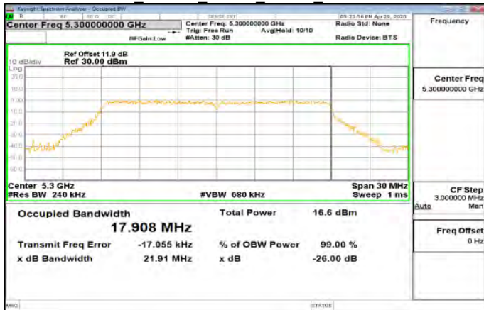
FCC 802.11n 20MHz Chain0 5300MHz
