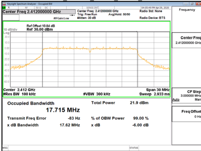
OBW 6dB 802.11n 20MHz Chain0 2412MHz
