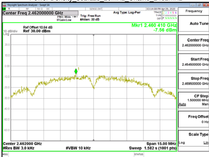
Power Density 802.11b 20MHz Chain0 2462MHz
