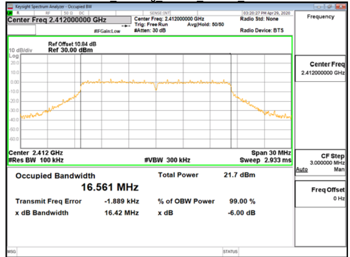
OBW 6dB 802.11g 20MHz Chain0 2412MHz
