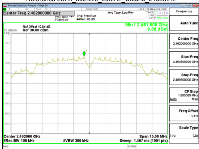
Reference Level 802.11b 20MHz Chain0 2462MHz
