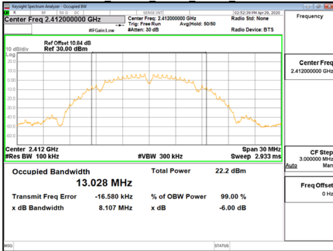
OBW 6dB 802.11b 20MHz Chain0 2412MHz
