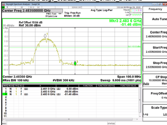
Band Edge 802.11b 20MHz Chain0 2462MHz
