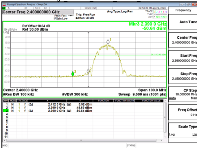
Band Edge 802.11b 20MHz Chain0 2412MHz
