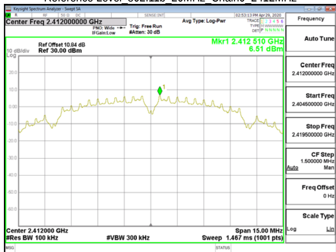
Reference Level 802.11b 20MHz Chain0 2412MHz
