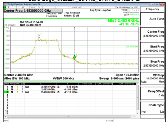
Band Edge 802.11n 20MHz Chain0 2462MHz
