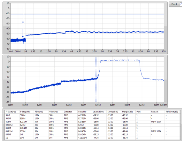
Band 5_LTE_3MHz_Nss1,QPSK_1TX 825.5MHz_QPSK_RB 1,#RB L
