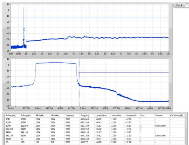
Band 5_LTE_10MHz_Nss1,QPSK_1TX 844MHz_QPSK_RB 1,#RB H
