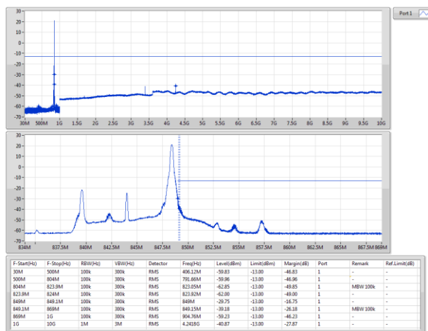
Band 5_LTE_10MHz_Nss1,QPSK_1TX 844MHz_QPSK_RB 1,#RB H
