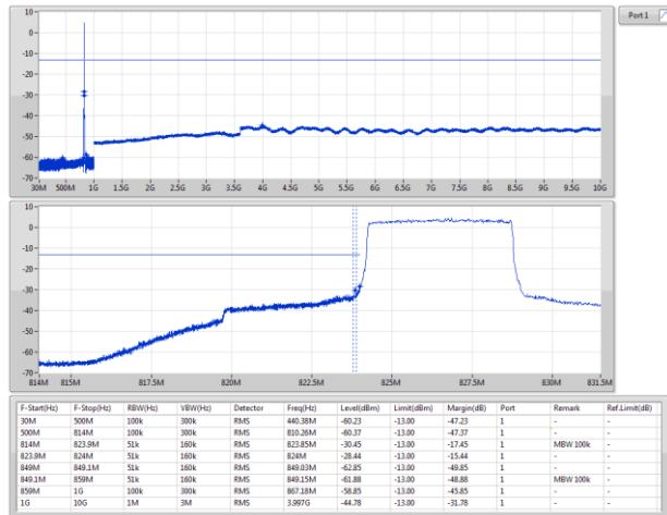
Band 5, LTE_5MHz_Nss1,QPSK_1TX 826.5MHz_QPSK_RB 1,#RB L
