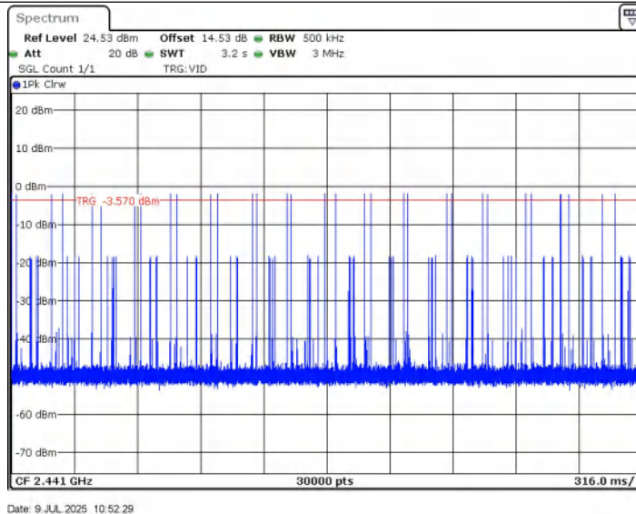
2DH3_Ant1_Hop
