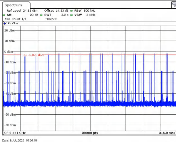
3DH3_Ant1_Hop
